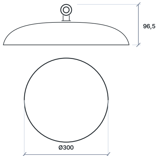
SHEMATSKI PRIKAZ / MJERE U mm
